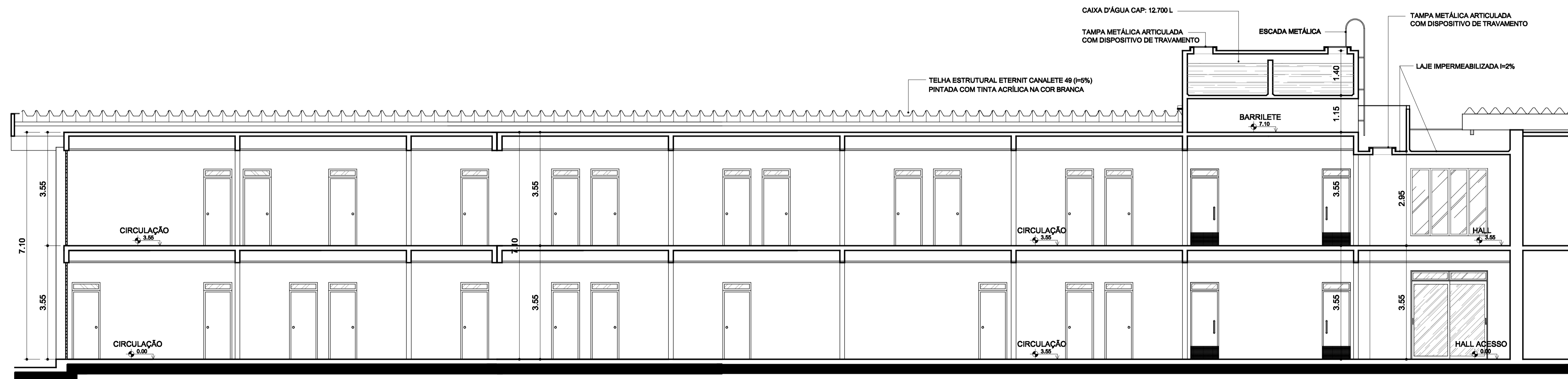
CORTE BB
