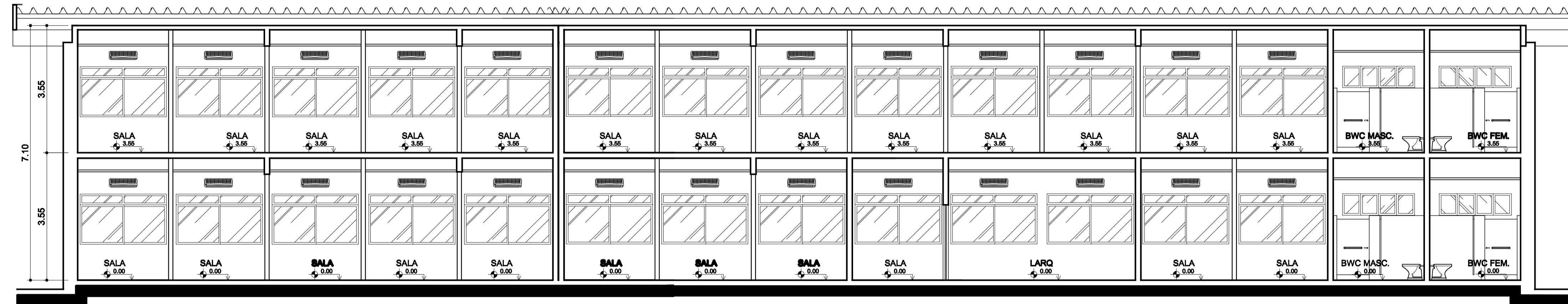
CORTE AA
