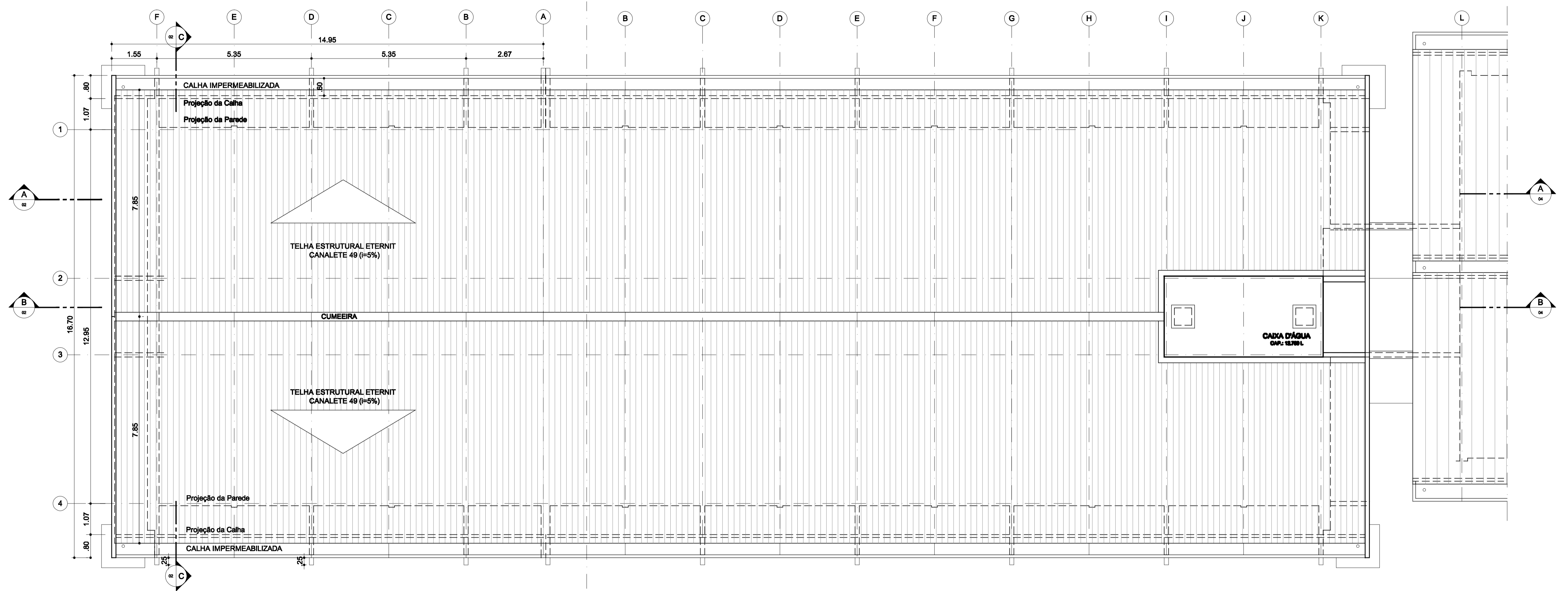
PLANTA DE COBERTA
