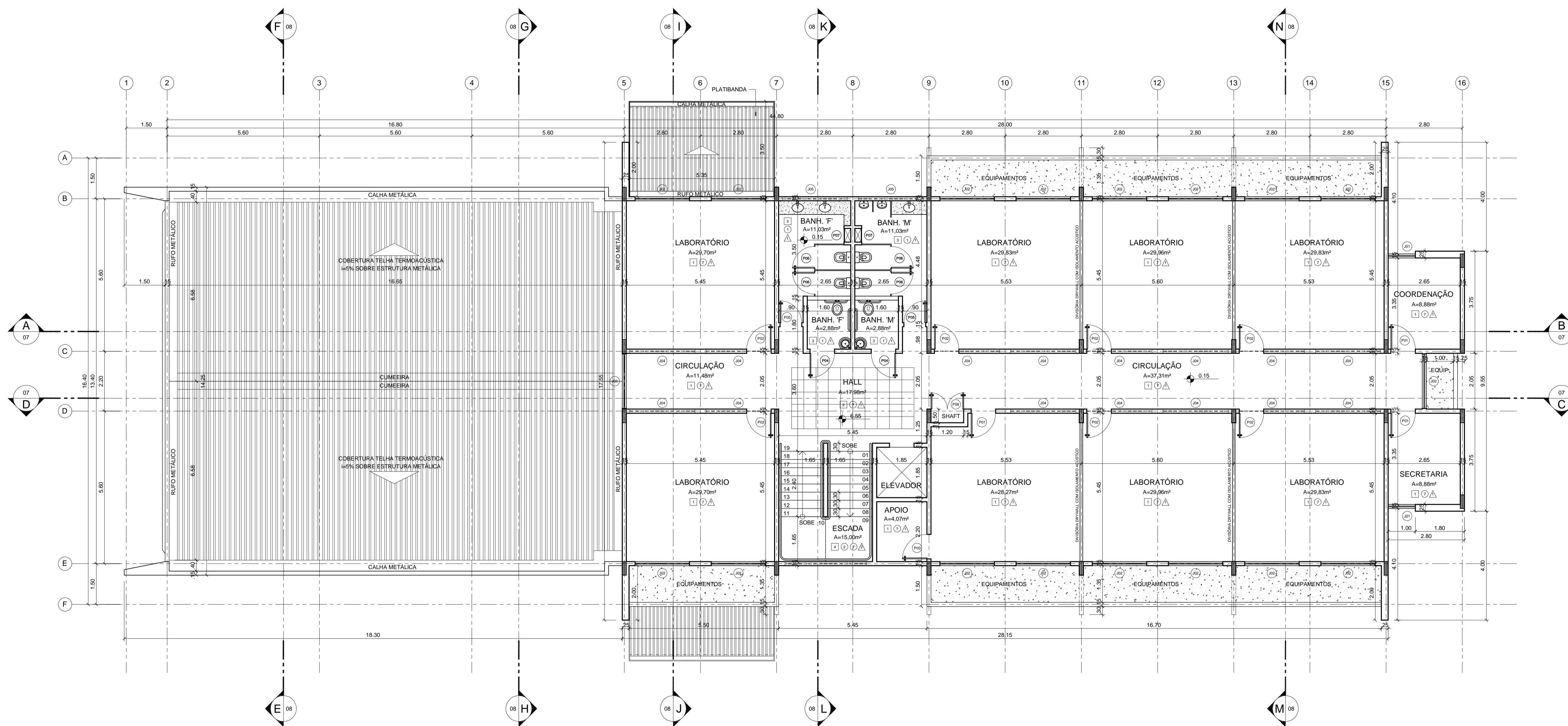
PLANTA BAIXA-PAV. 03 ESCALA 1/75
